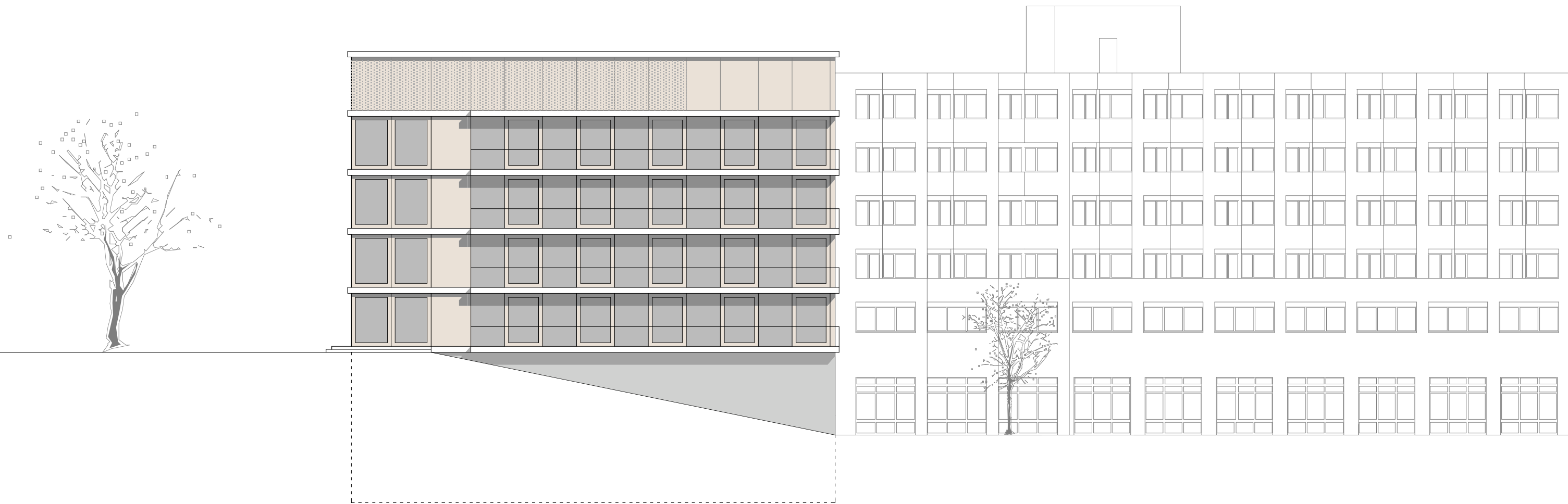
Ansicht Süd 1:200
